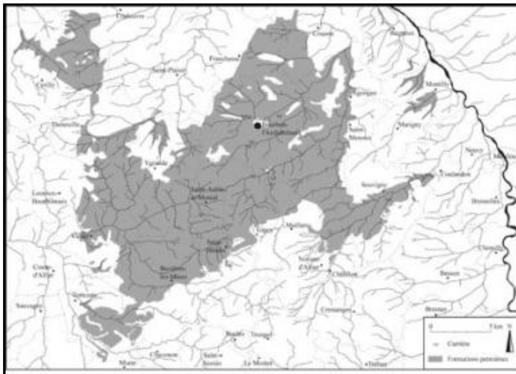
Fig. 1. Carte des affleurements de grès permien dans le centre de l'Allier et des carrières reconnues (A. Fourvel).
