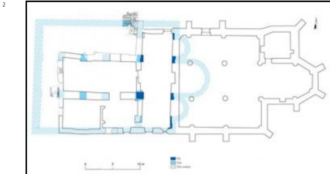
Fig. 1. État du XII e siècle restitué (dessin J. Mercier, CEM).
