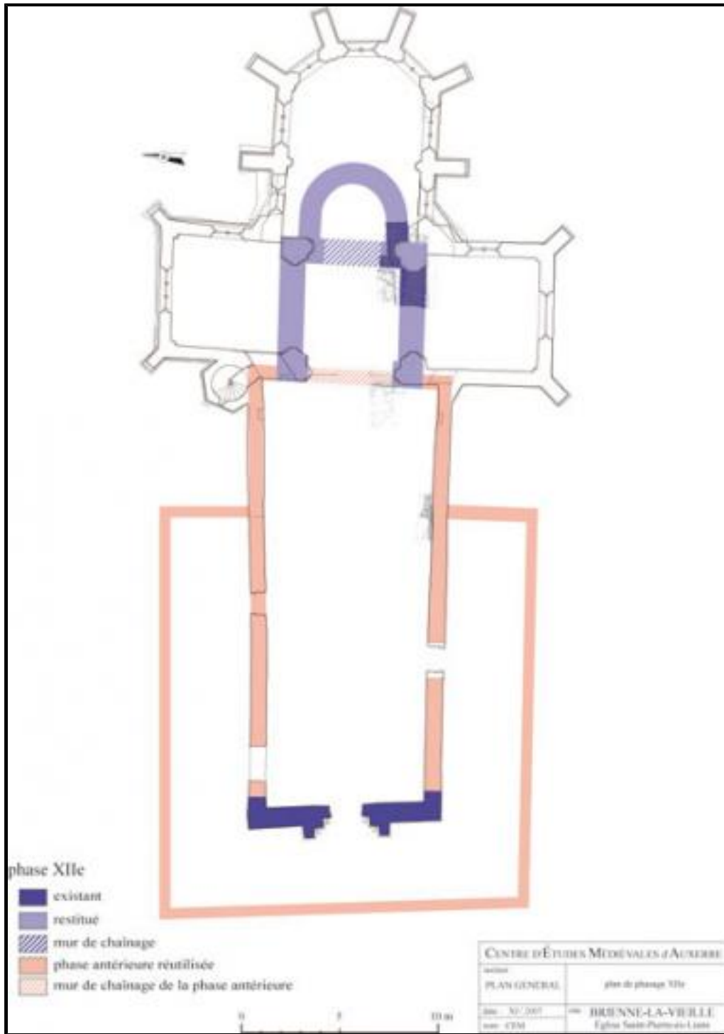
Fig. 1 - Saint-Pierre-ès-liens. Brienne-la-Vieille, plan de phasage XII e siècle.
