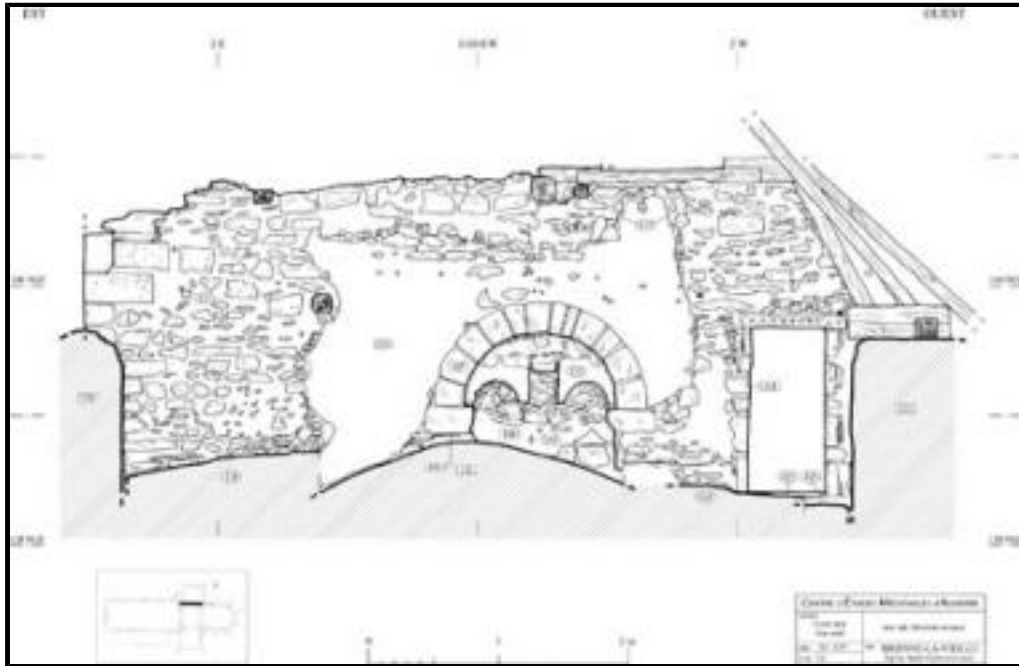
Fig. 2 - Brienne-la-Vieille, mur nord, élévation est/ouest
