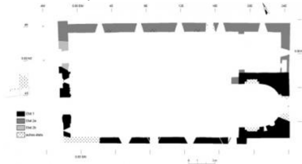
Saint-Père, église Saint-Pierre. Plan de phasage (dessin G. Fèvre - CEM).
