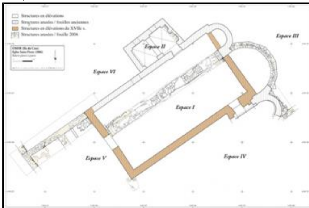
Fig. 2 - Église Saint-Pierre d'Osor, plan pierre à pierre (del. D. Vuillermoz, d'après équipe de fouilles).
